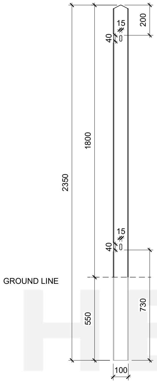
SCALE 1:15
